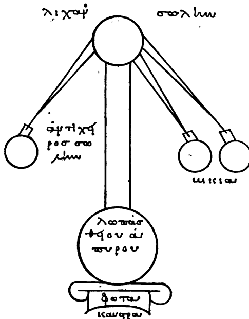
FIGURE 15. — Alambic à trois récipients (tribikos). Réduction aux 2/3.
